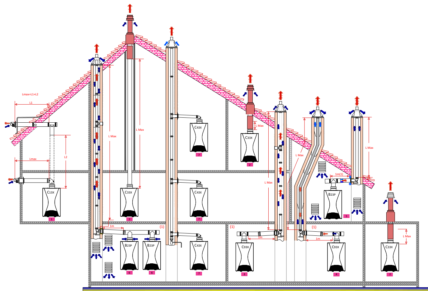
(1) На 1 метр увеличение дымохода по горизонтали длина вертикального дымохода уменьшается на 1,2 метра.
