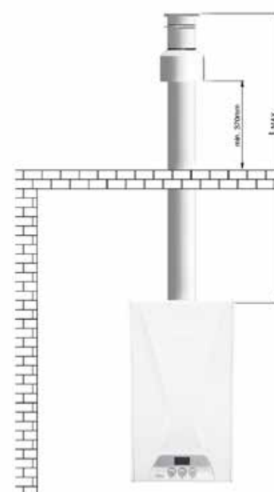
Вертикальная система дымоудаления (Lмакс. без колена: 4 м, 60/100) (Lмакс. без колена: 8 м, 80/125)
