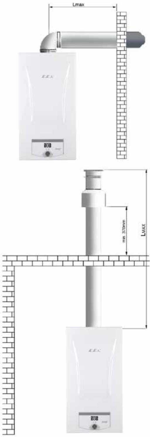
Горизонтальное исполнение дымохода: макс. длина L с одним коленом: 4 м, 60/100
