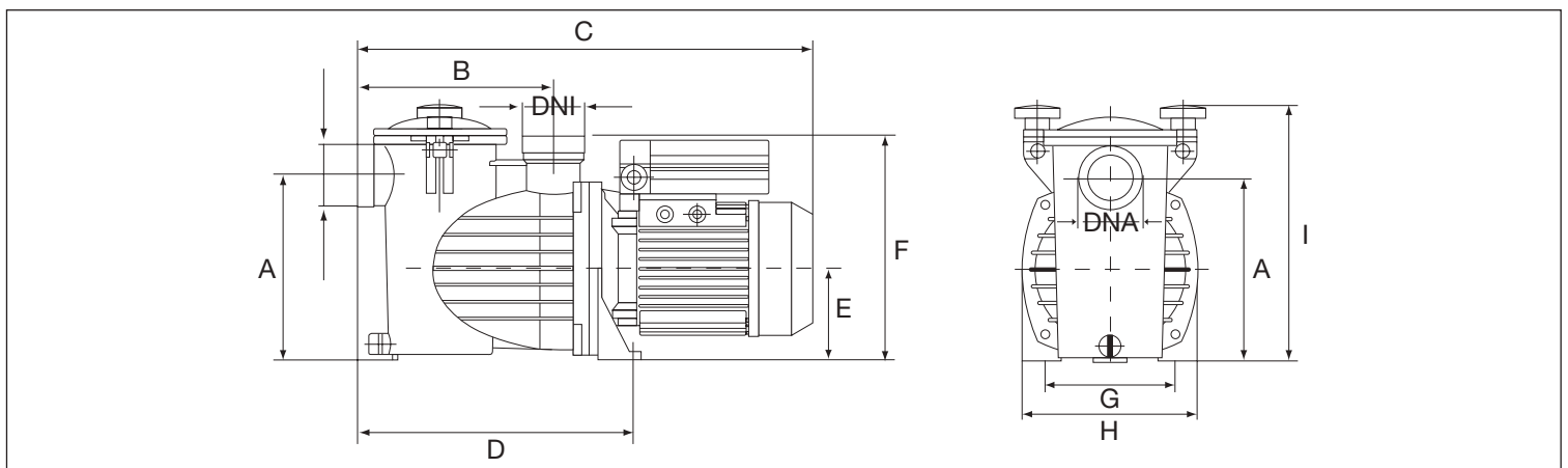
РАЗМЕРЫ SWS
