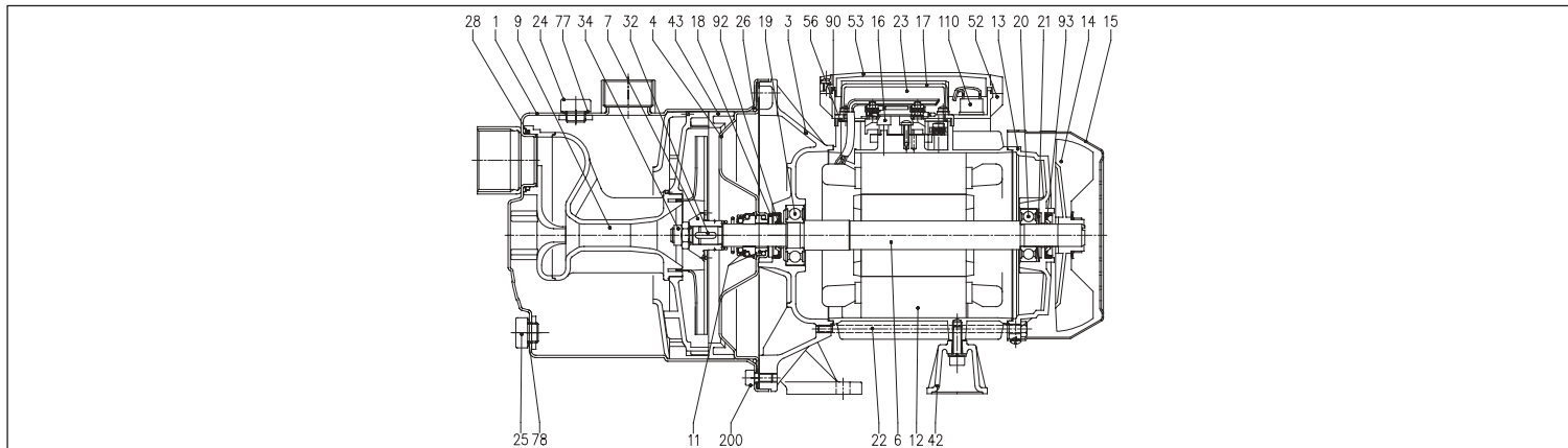
РАЗРЕЗ JEX
