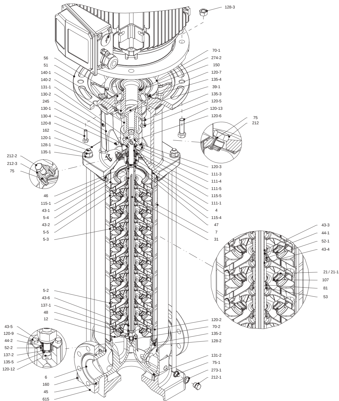
Насос с одиночным шариковым подшипником от 37 кВт
