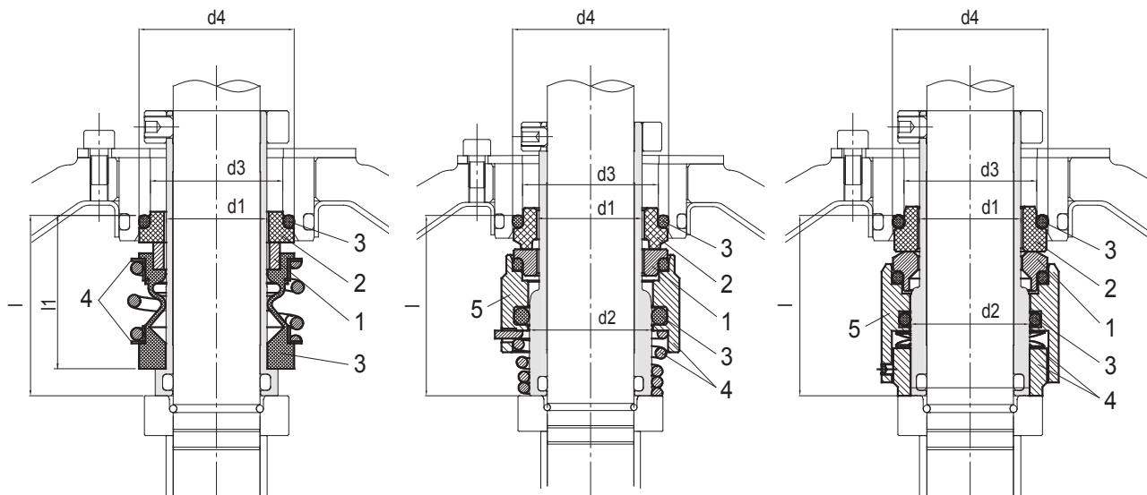
до 16 бар Картриджное несбалансированное уплотнение
