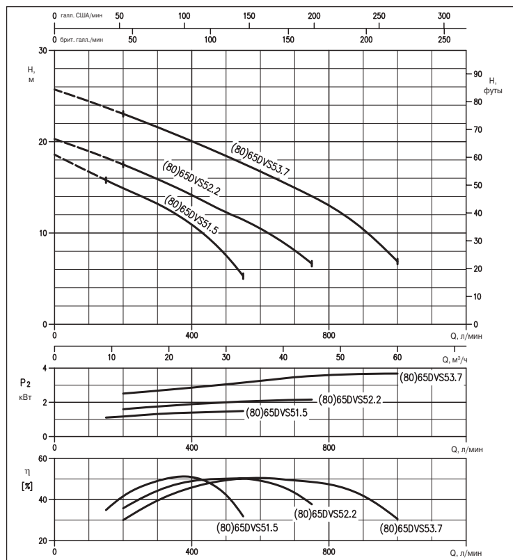
ГРАФИК РАБОЧИХ ХАРАКТЕРИСТИК (по ISO 9906, Приложение А)
