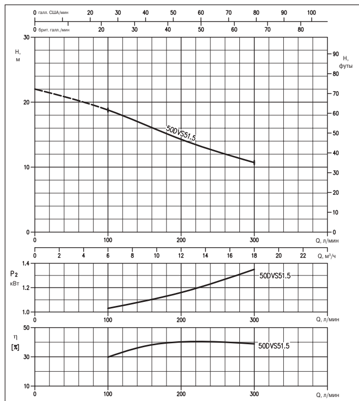
ГРАФИК РАБОЧИХ ХАРАКТЕРИСТИК (по ISO 9906, Приложение А)
