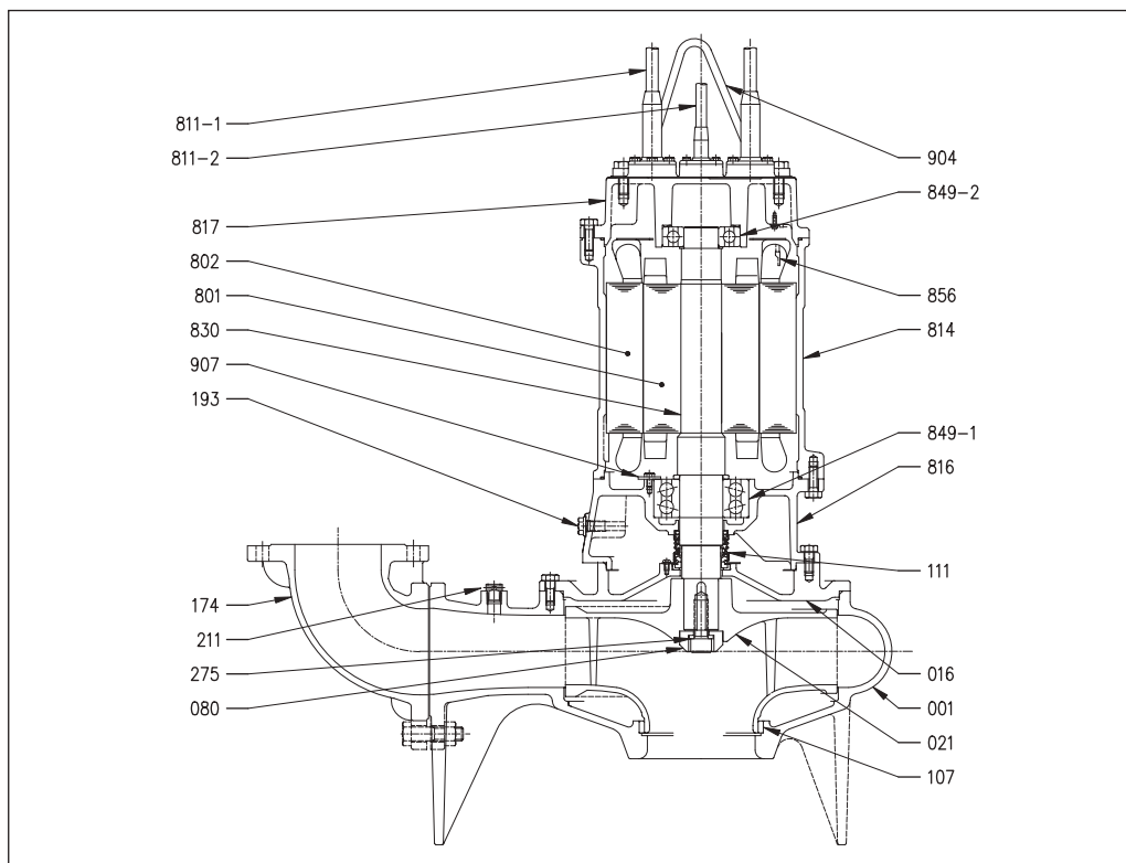
МОДЕЛЬ 100 (150) DML в разрезе (11 - 22 кВт)
