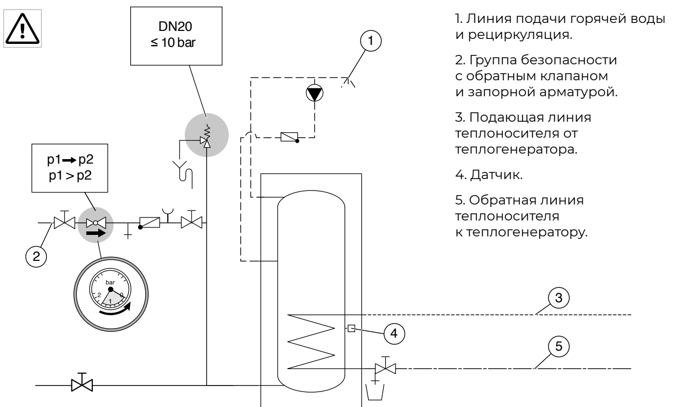
Рис. 10. Схема обвязки.
