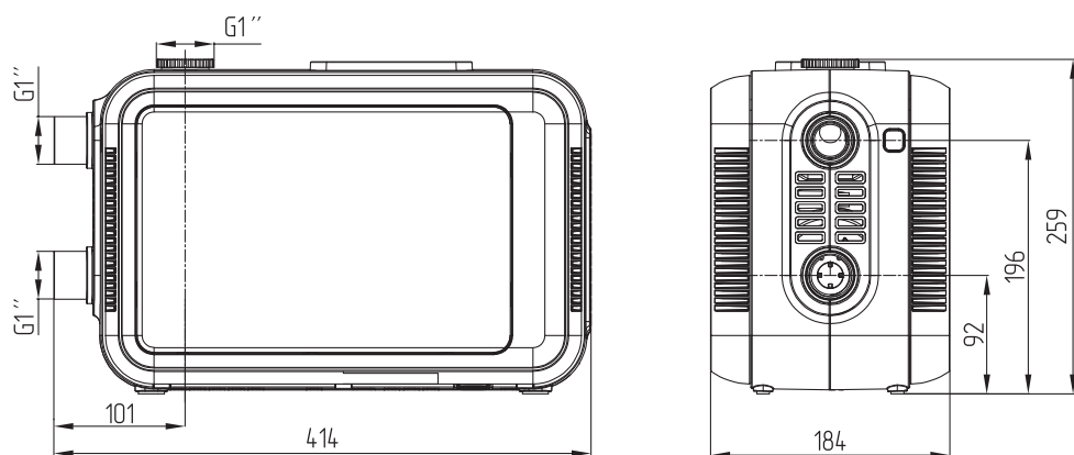
Рис. 4 Габаритные размеры насосной станции ZOTA LaScala
