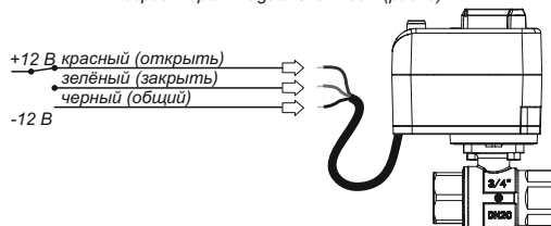
Электрическая схема подключения крана с электроприводом серии Neptun Bugatti Click 12B (рис. 4)
