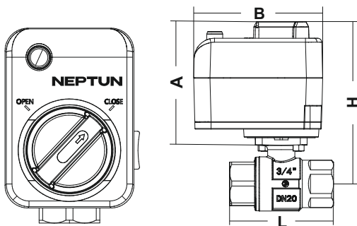
Габаритные размеры (рис. 1)
