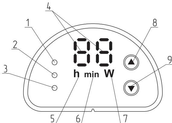
Рис.7 Панель управления
