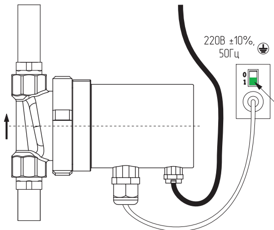
Рис.5 Электроподключение насоса
