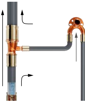
Рис. 06-5 Принцип работы кольцевого трубопровода с изогнутыми тройником РЕХАУ RX+
