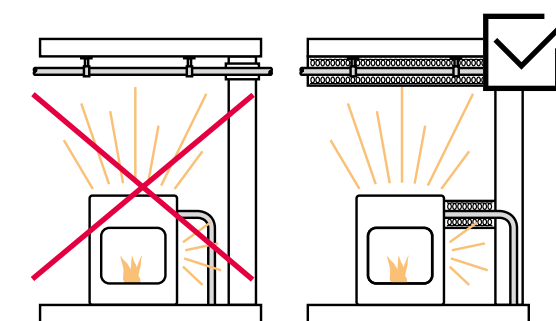
Рис. 37-3 Защита от перегрева
