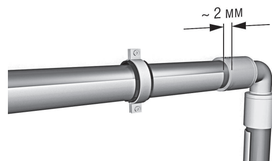
Рис. 6 Фиксирующий желоб должен не доходить до подвижной гильзы на 2 мм
