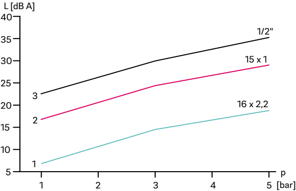
Рис. 22-3 Результат Протокол испытания Института Фраун-гофера: сравнение материалов труб
