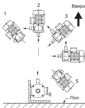
Рис. 4 Положения насоса
