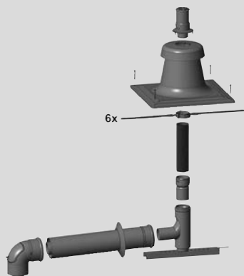
Комплект с концентрическим подключением к дымоходу в шахте для режима подачи воздуха для горения из атмосферы
