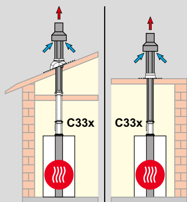
Концентрический вертикальный проход через наклонную или плоскую кровлю
