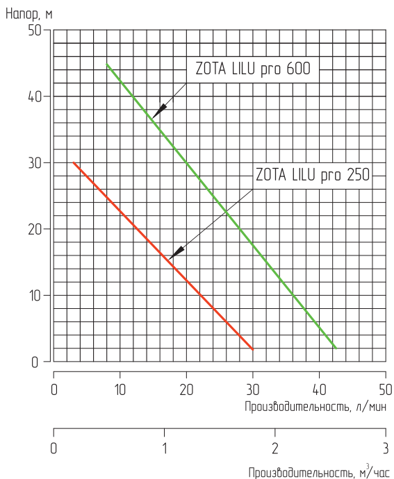
Рис. 1 Расходно-напорные характеристики
