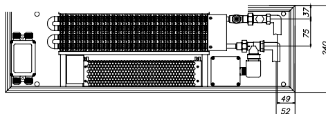
ЕКQ.240.90, ЕКQ.240.110, ЕКQ.240.150, вид сверху
