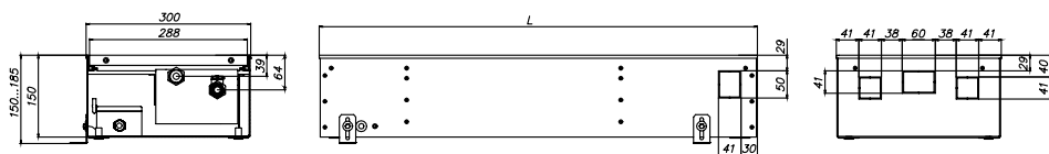
ЕКQ.300.150, вид сбоку
