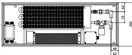
ЕКQ.300.90, вид сбоку
