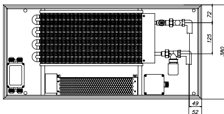
ЕКQ.380.90, ЕКQ.380.110, ЕКQ.380.150, вид сверху
