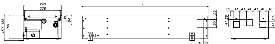
ЕКQ.240.150, вид сбоку
