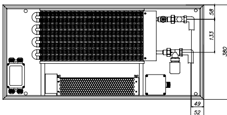
ЕКQ.380.75 вид сбоку
