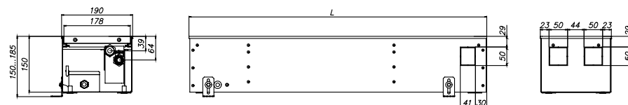
ЕКQ.190.150, вид сбоку
