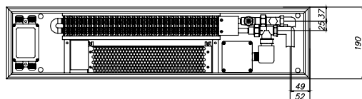
ЕКQ.190.90, ЕКQ.190.110, ЕКQ.190.150, вид сверху
