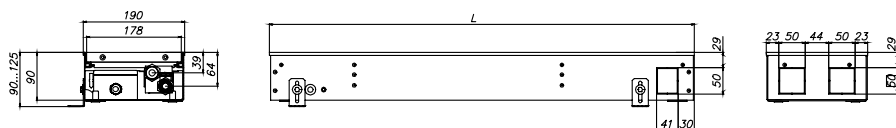
ЕКQ.190.110, вид сбоку
