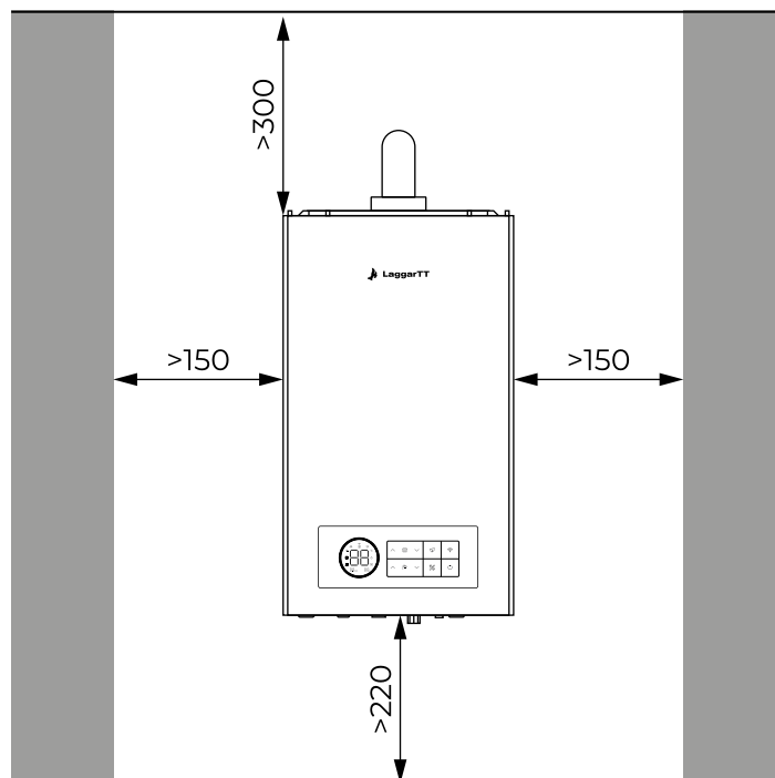
Рис. 44. Рекомендуемые расстояния для монтажа.
