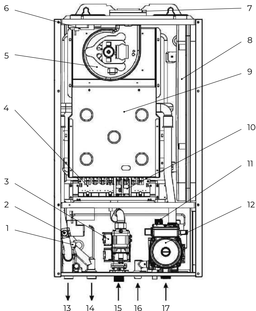
Рис. 4. Общая схема котлов B30 18 Н (Wi-Fi), 24 Н (Wi-Fi).
