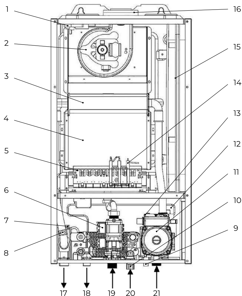
Рис. 2. Общая схема котлов B30 18 C (Wi-Fi), 24 C (Wi-Fi).
