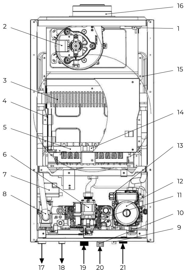
Рис. 3. Общая схема котлов B30 28 C (Wi-Fi), 32 C (Wi-Fi), 36 C (Wi-Fi).
