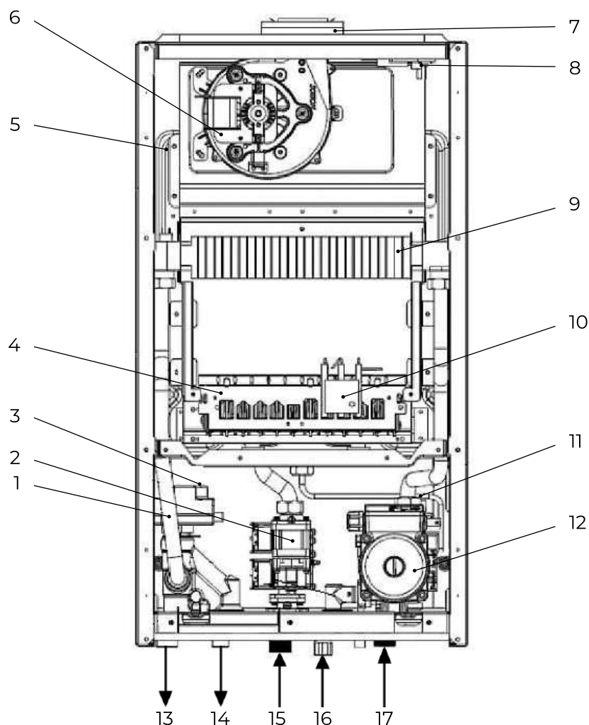
Рис. 5. Общая схема котлов B30 28 Н (Wi-Fi), 32 Н (Wi-Fi), 36 Н (Wi-Fi).
