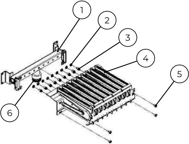
Рис. 39. Газовая горелка.
