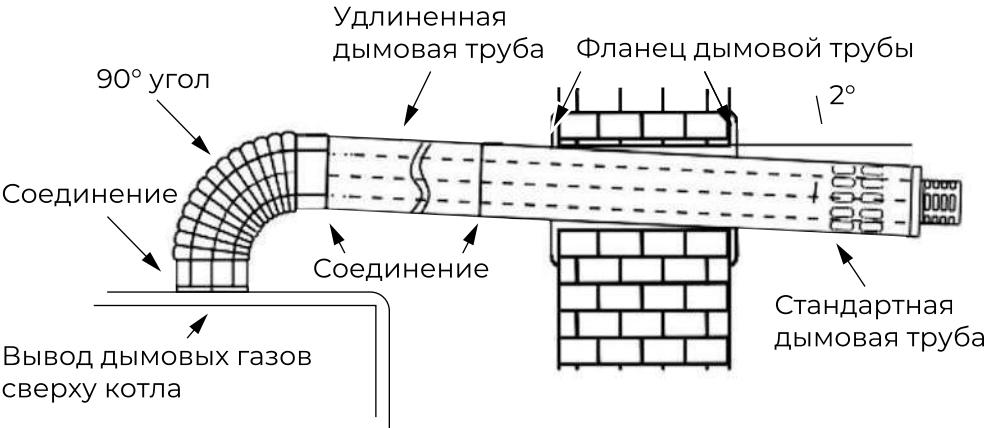
Рис. 45. Пример монтажа схемы C12.
