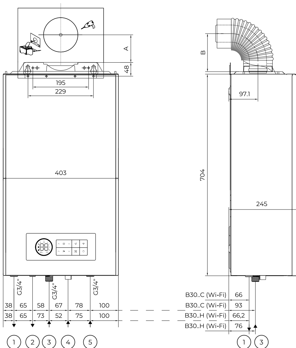
Рис. 42. Монтажные размеры В30 18 С/Н (Wi-Fi), В30 24 С/Н (Wi-Fi).
