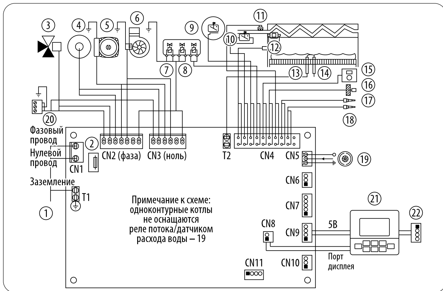
Рис. 46. Электрическая схема.
