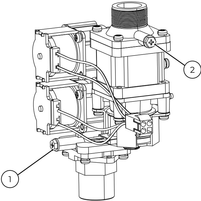
Рис. 40. Газовый клапан.
