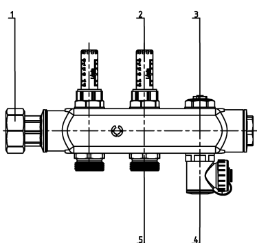
Подающая балка артикул 1404300xx
