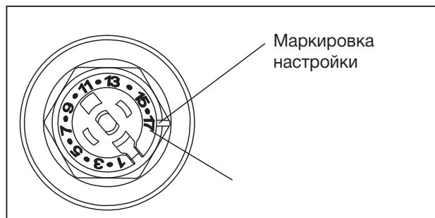
Рис. 7 Преднастройка расхода
