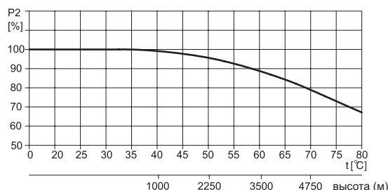
Рис. 16 Максимальная мощность двигателя зависит от температуры окружающей среды и высоты над уровнем моря
