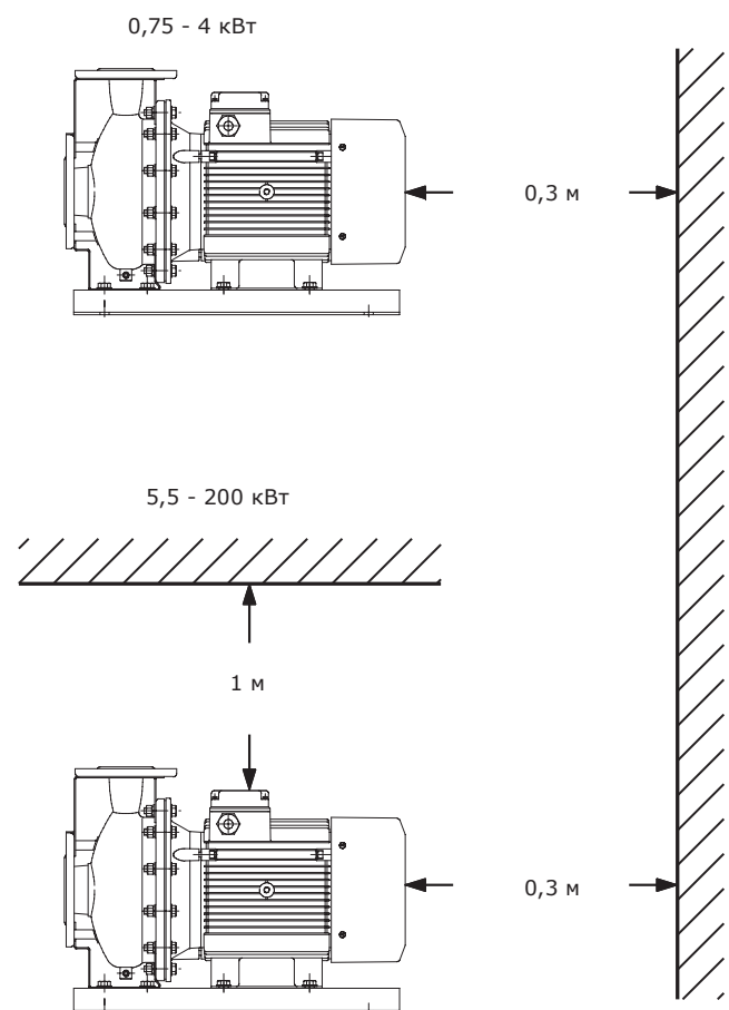
Рис. 5 Пространство за двигателем
