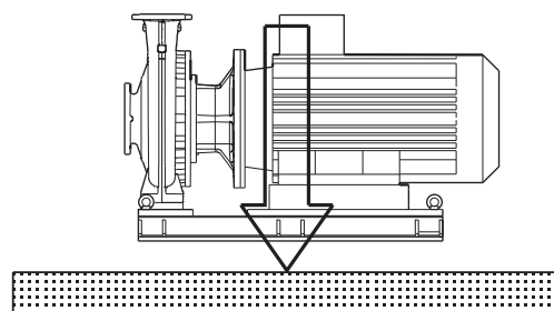
Рис. 8 Подходящий фундамент
