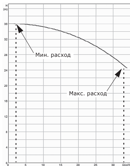
Рис. 18 Пример с указанием минимального и максимального расхода
