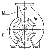
Рис. 15 Сливная пробка и пробка для выпуска воздуха (местоположение пробок может отличаться от указанного)
