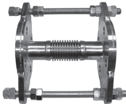
Рис. 14 Вибровставка с металлическим сильфоном и ограничительными стяжками
