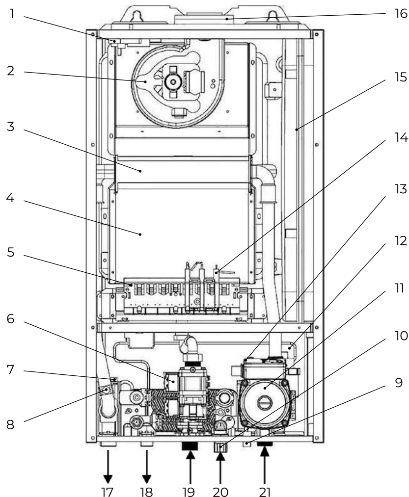
Рис. 2. Общая схема котлов В30 18 С, 24 С.
