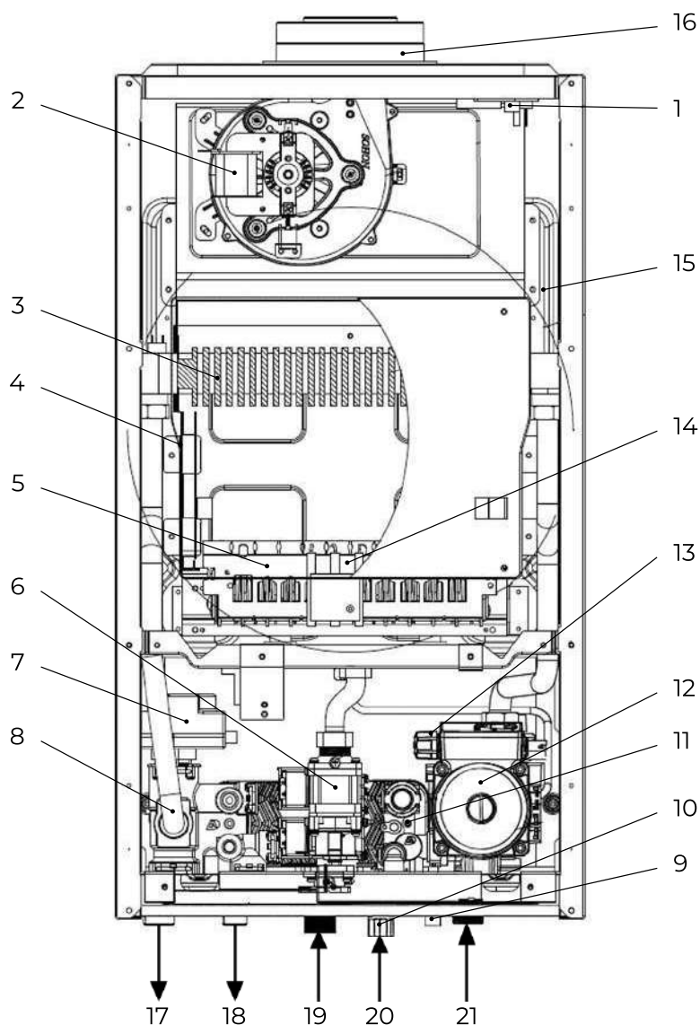
Рис. 3. Общая схема котлов V30 28 C, 32 C, 36 C.
