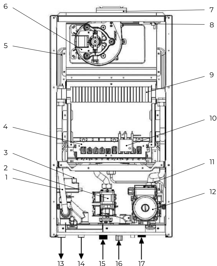
Рис. 5. Общая схема котлов B30 28 Н, 32 Н, 36 Н.
