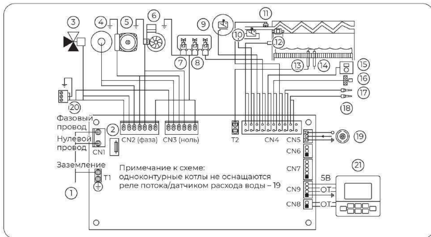
Рис. 31 . Электрическая схема.
