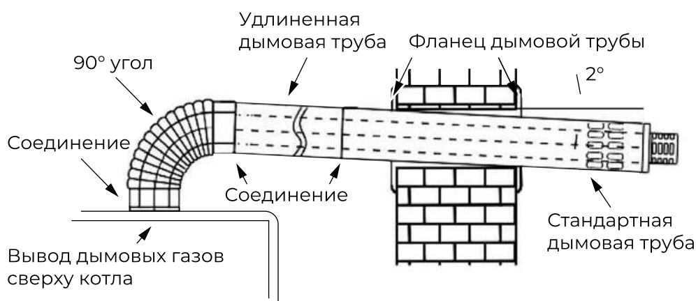
Рис.30. Пример монтажа схемы C12.
