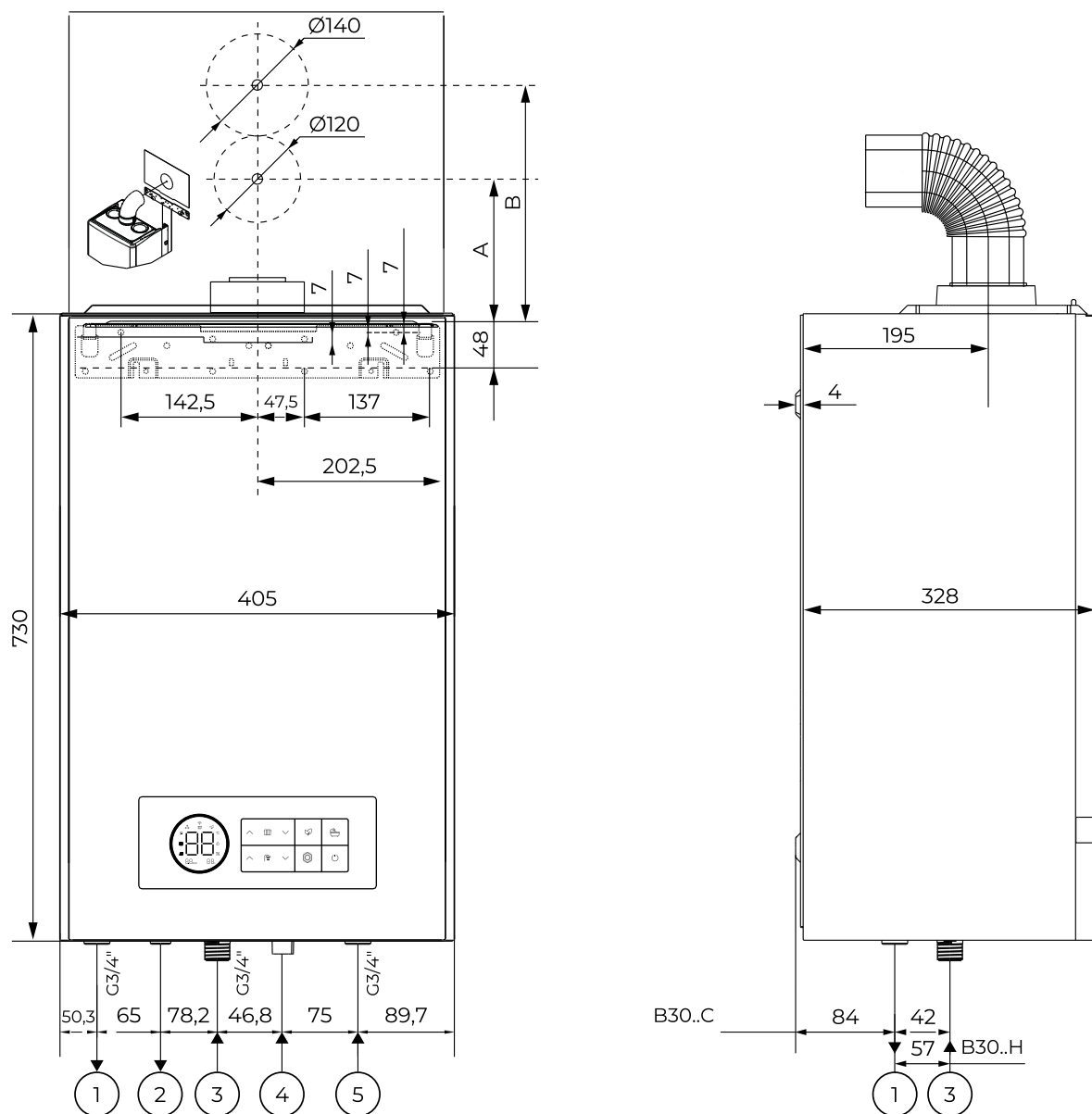
Рис. 28. B30 28 C/H, B30 32 C/H, B30 36 C/H.
