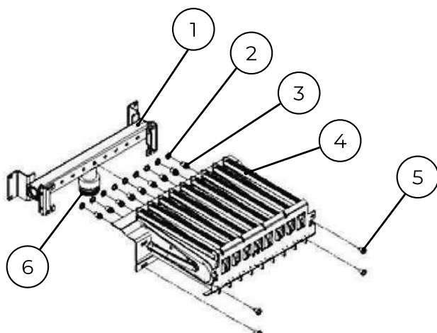
Рис. 24. Газовая горелка.
