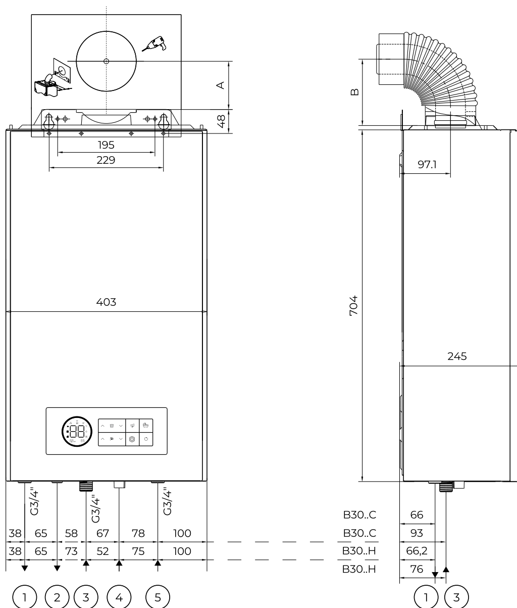
Рис. 27. Монтажные размеры B30 18 C/H, B30 24 C/H.
