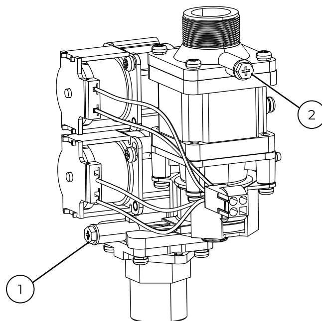
Рис. 25. Газовый клапан.
