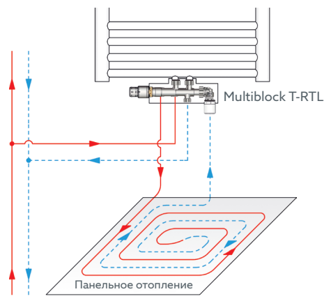
Пример системы Multiblock T – RTL с регулируемым контуром панельного отопления
