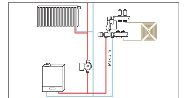
Рис. 1-4 Схема подключения с первичным циркуляционным насосом в котле
