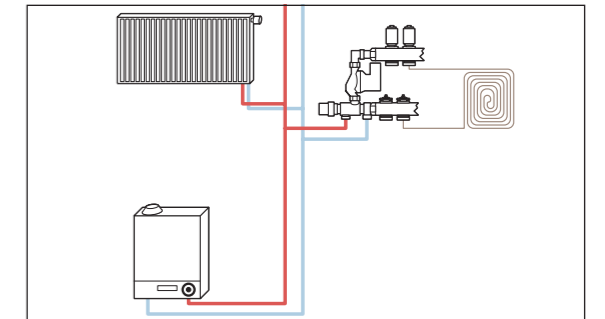
Рис. 1-3 Схема подключения с первичным циркуляционным насосом в котле
