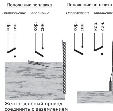
Рис. 6 Электрическое подключение KR 1
