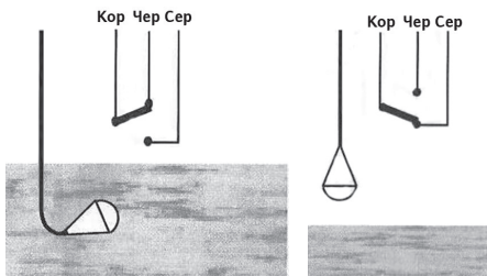
Рис. 5 Электрическое подключение MS 1 и MS M2
