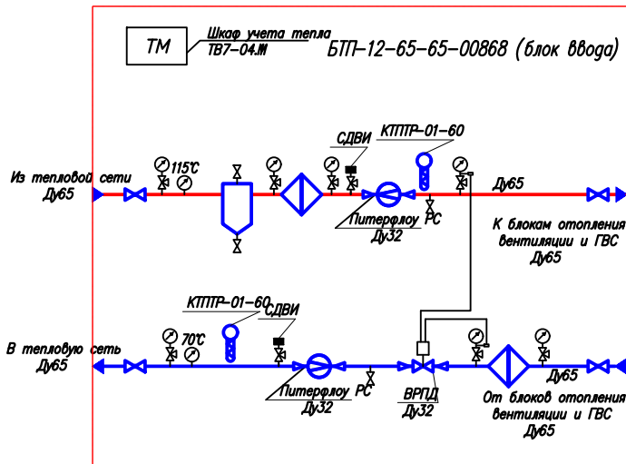
БТП-12-65-65-00868 (блок ввода)
