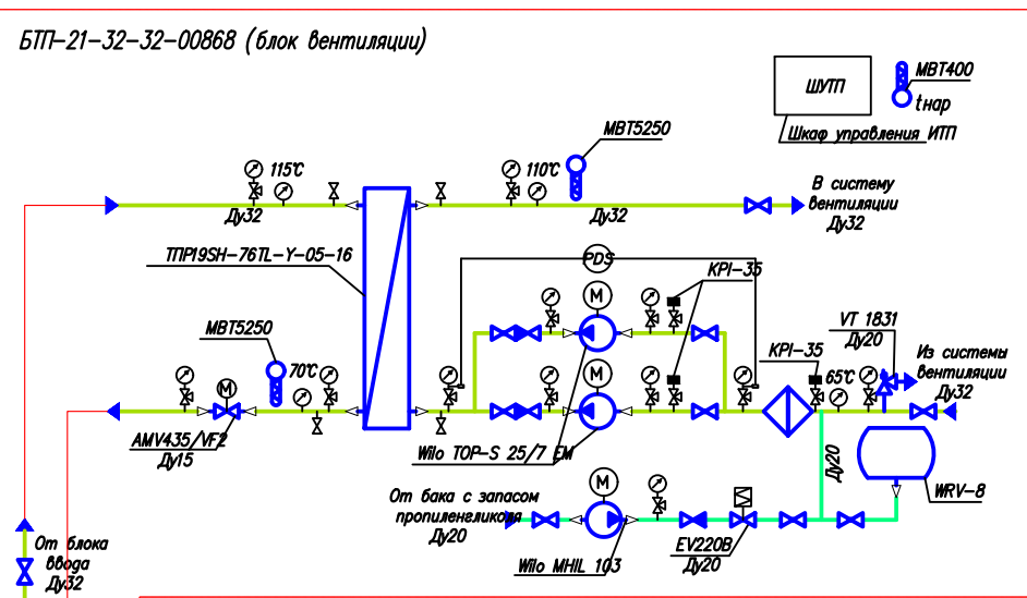
Принципиальная схема блочного теплового пункта БТП-12-65-65-00868
